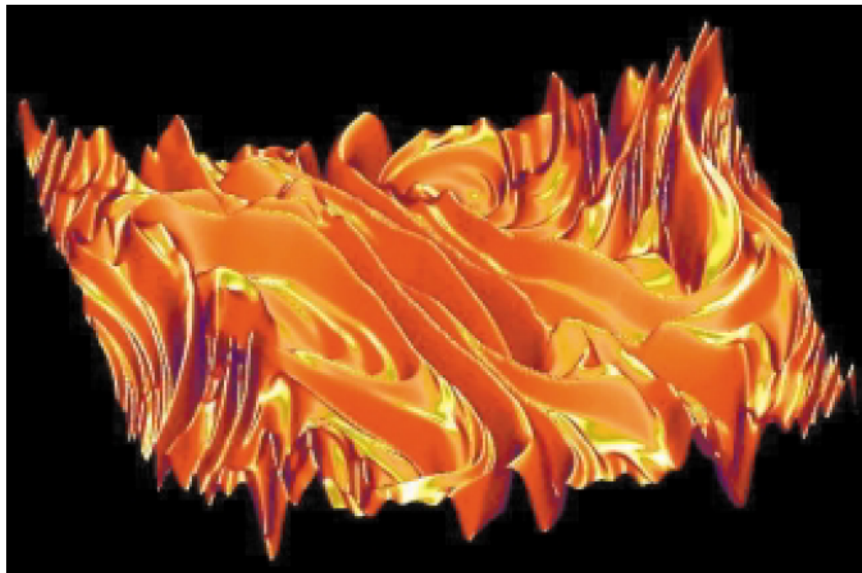
上：2次元乱流の可視化
