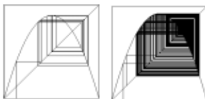
ロジスティクス写像を何回も合成したときの点の動き
