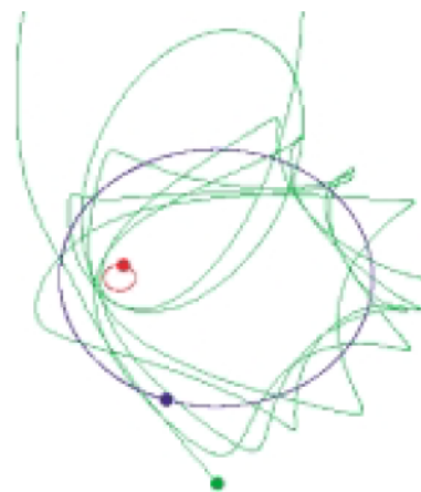
3体問題で、複雑な軌道がうまれるこるメカニズム
