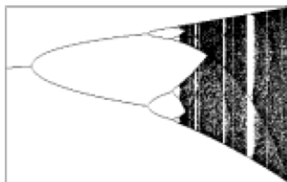
\alpha の変化でカオスが生じる様子
